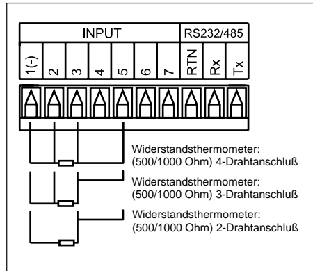
Abbildung 2-12. Anschluß eines Pt 500 oder Pt 1000
