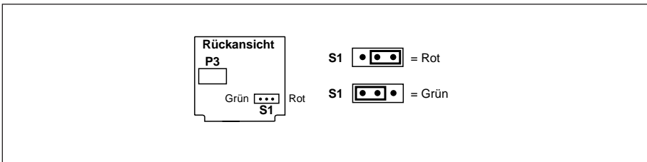
Abbildung 2-25. Einstellung der Farbe der zweiten Displayzeile, Modell i16D
