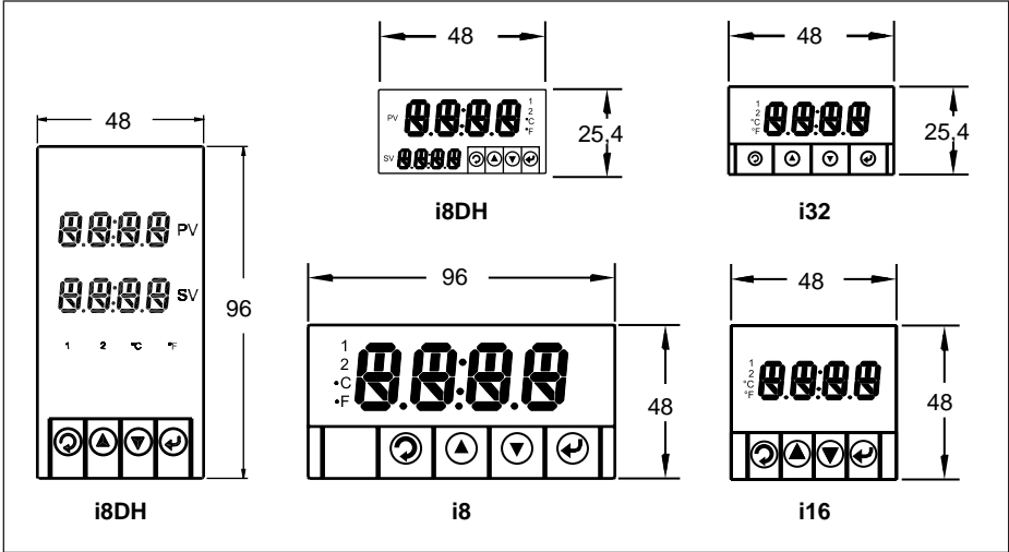
Abbildung 2-2. Frontplatte und Abmessungen
