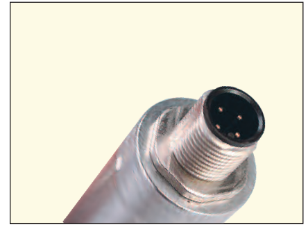
PXM459: M12-Steckverbinder Schutzart IP67, absolut; Schutzart IP65, relativ
