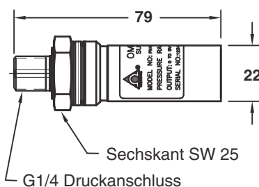
PXM409-Serie mit Druckbereichen bis 1 bar
